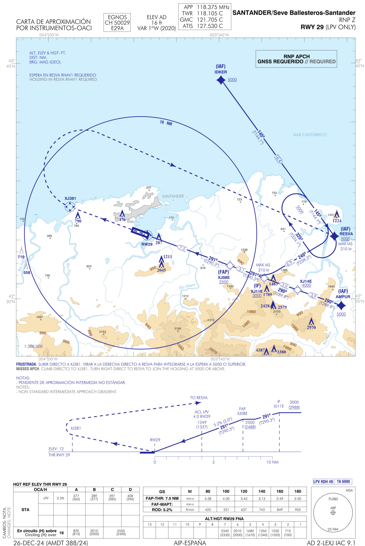
Figura 3.22: Aproximación por instrumentos a LEXJ RWY 29 procedimiento LPV [Fig27].
