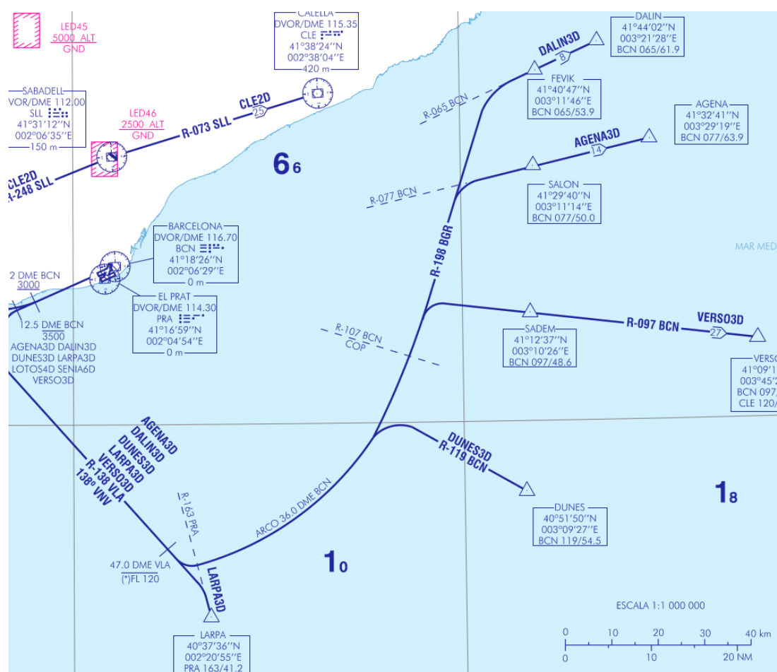
Figura 3.19: Extracto de SID convencional de la RWY 25R de LEBL [Fig26].
