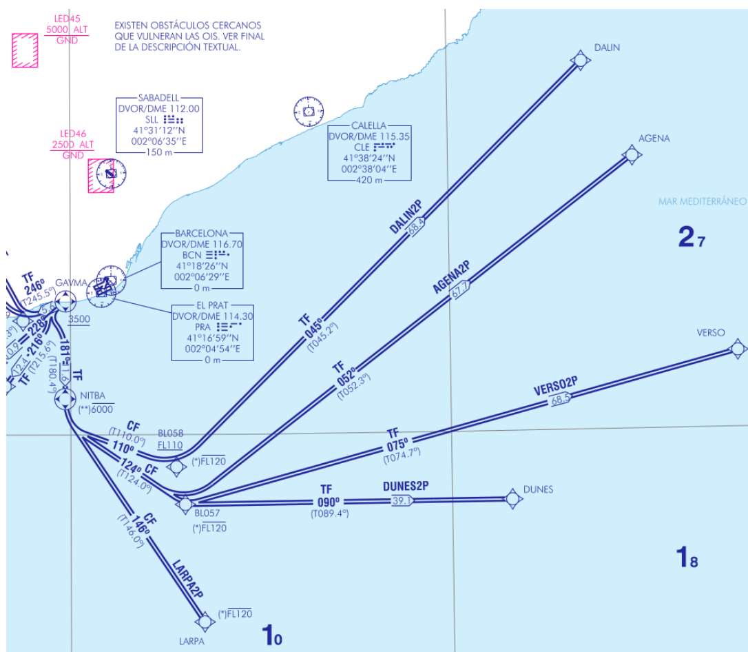
Figura 3.20: Extracto de SID P-RNAV de la RWY 25R de LEBL [Fig26].
